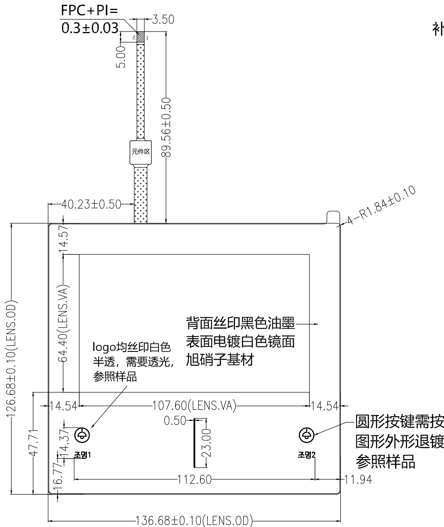
正面视图
