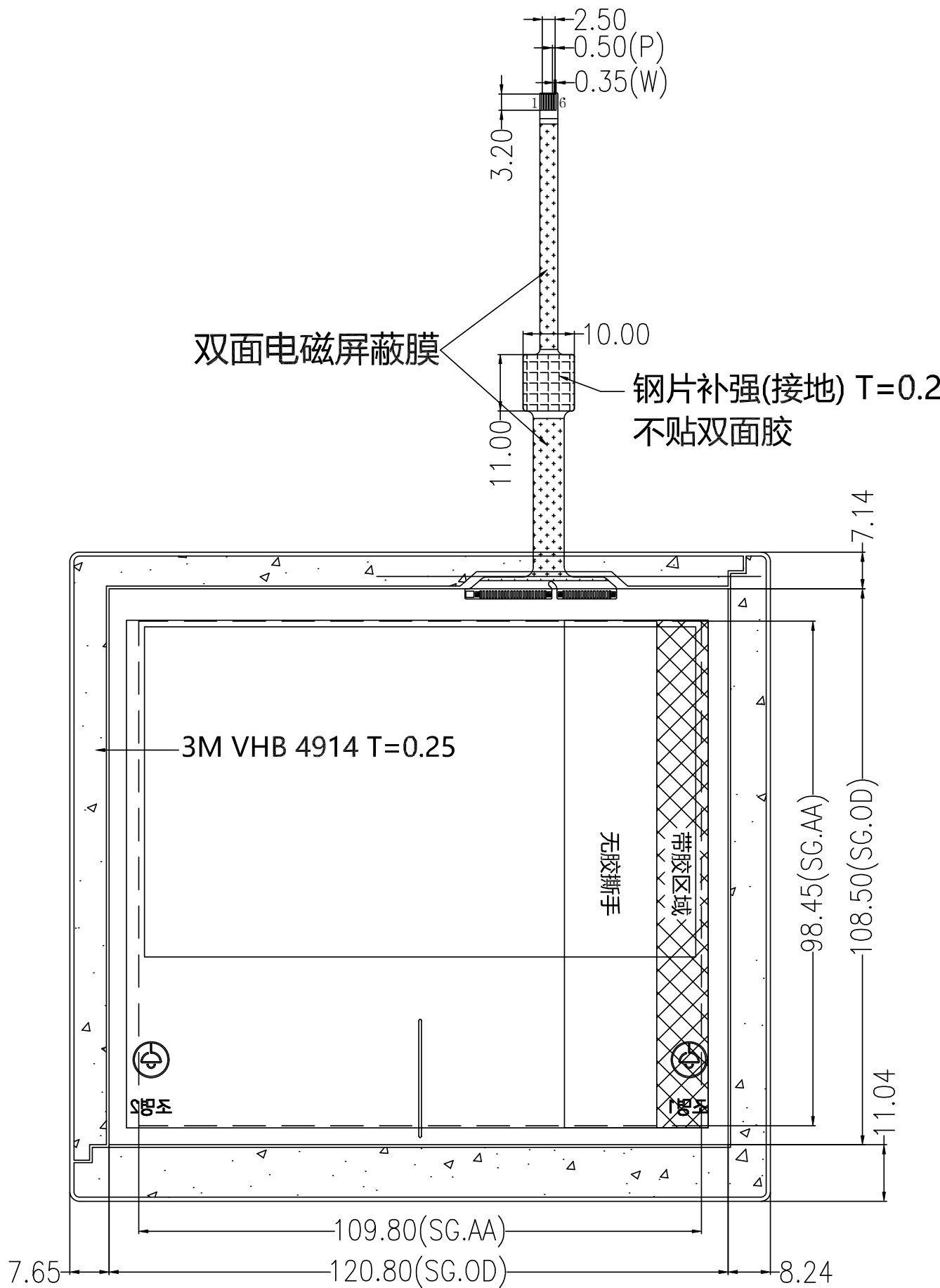
背面视图
